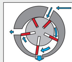
Vane motor
